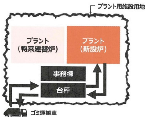
図-3 将来建替炉の建築スペース
